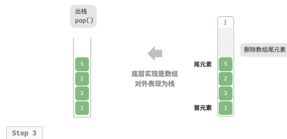
图 5-3 基于数组实现栈的入栈出栈操作
