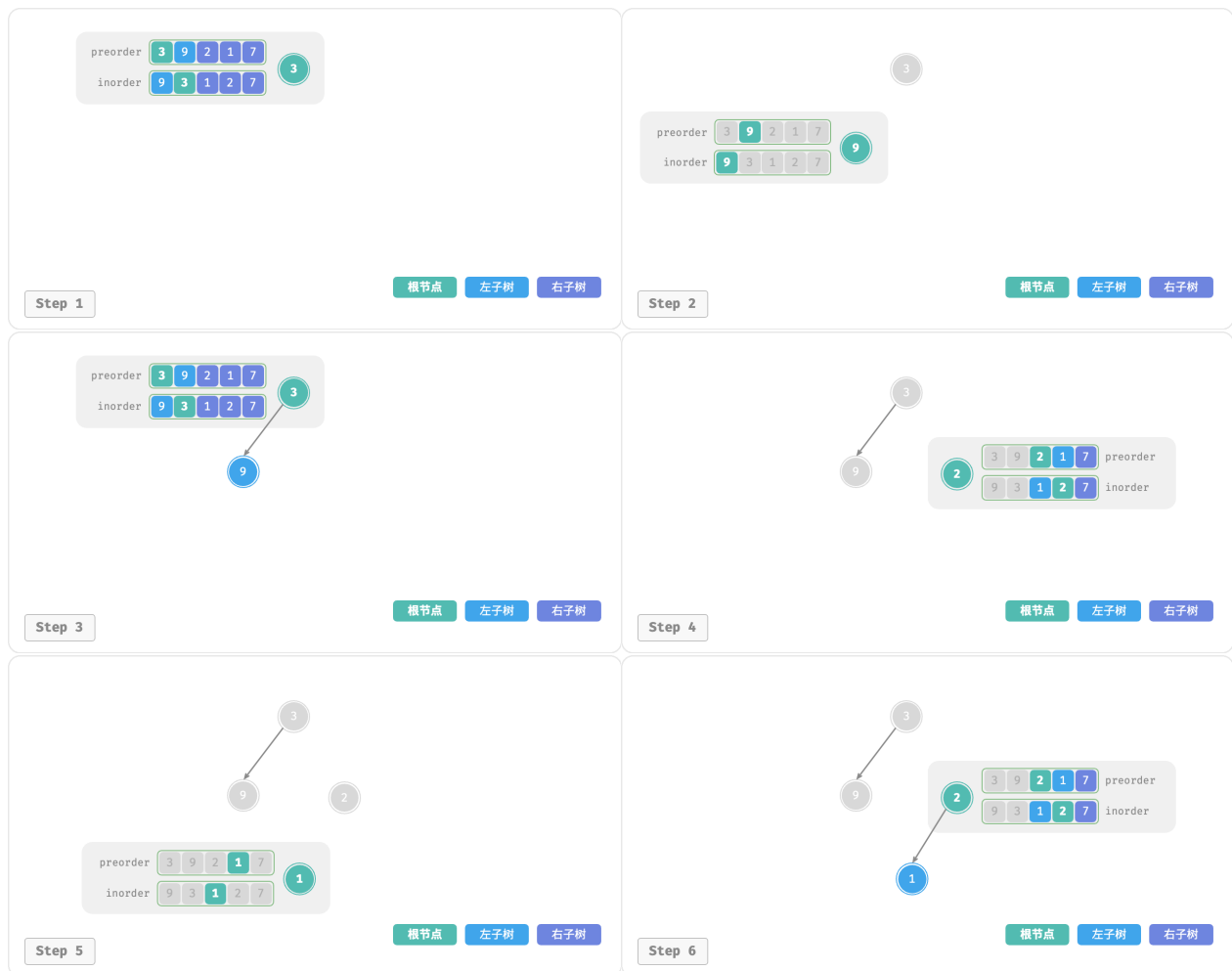
图 12-8 展示了构建二叉树的递归过程, 各个节点是在向下“递”的过程中建立的, 而各条边(引用)是在向上“归”的过程中建立的。
