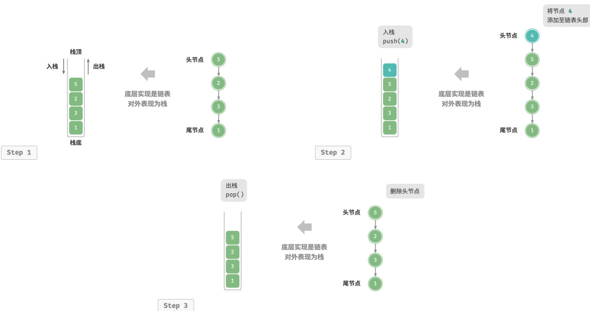
图 5-2 基于链表实现栈的入栈出栈操作
