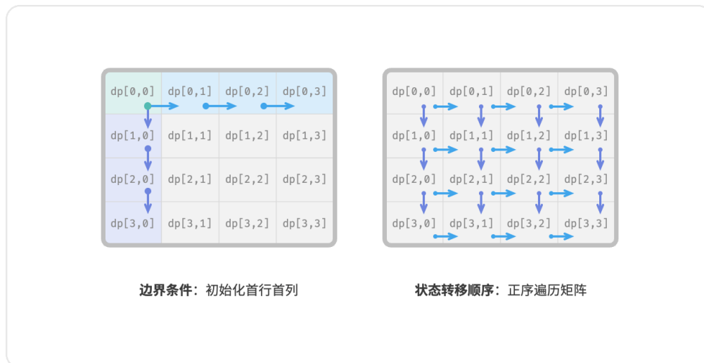
图 14-13 边界条件与状态转移顺序
