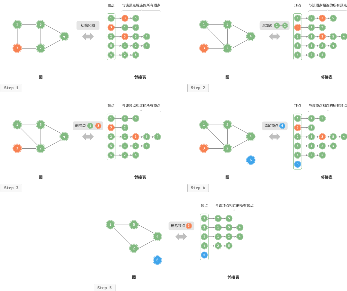
图 9-8 邻接表的初始化、增删边、增删顶点
