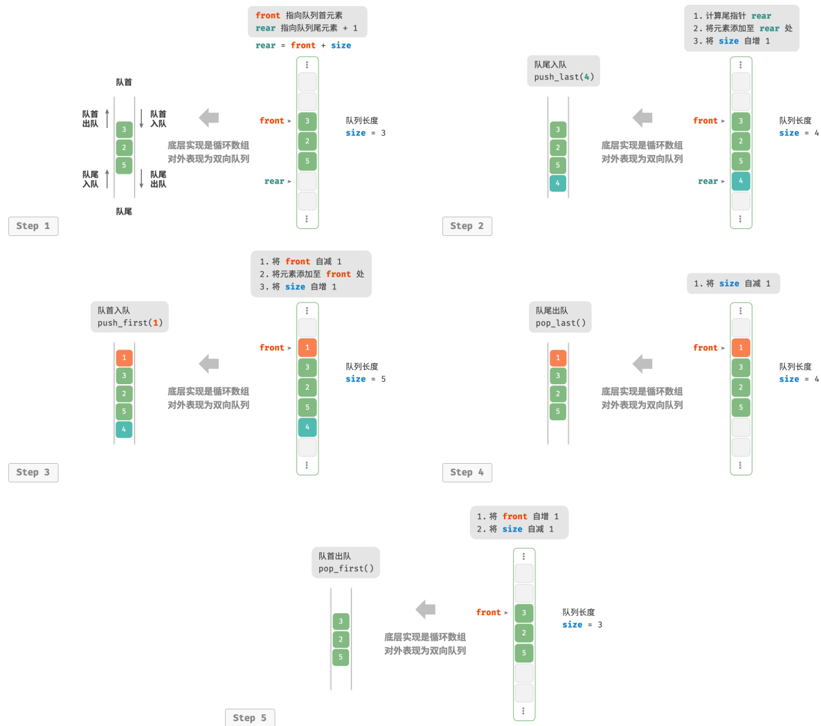
图 5-9 基于数组实现双向队列的入队出队操作
