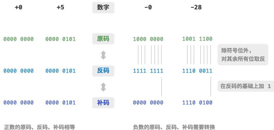
图 3-4 原码、反码与补码之间的相互转换
