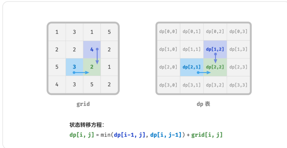
图 14-12 最优子结构与状态转移方程
