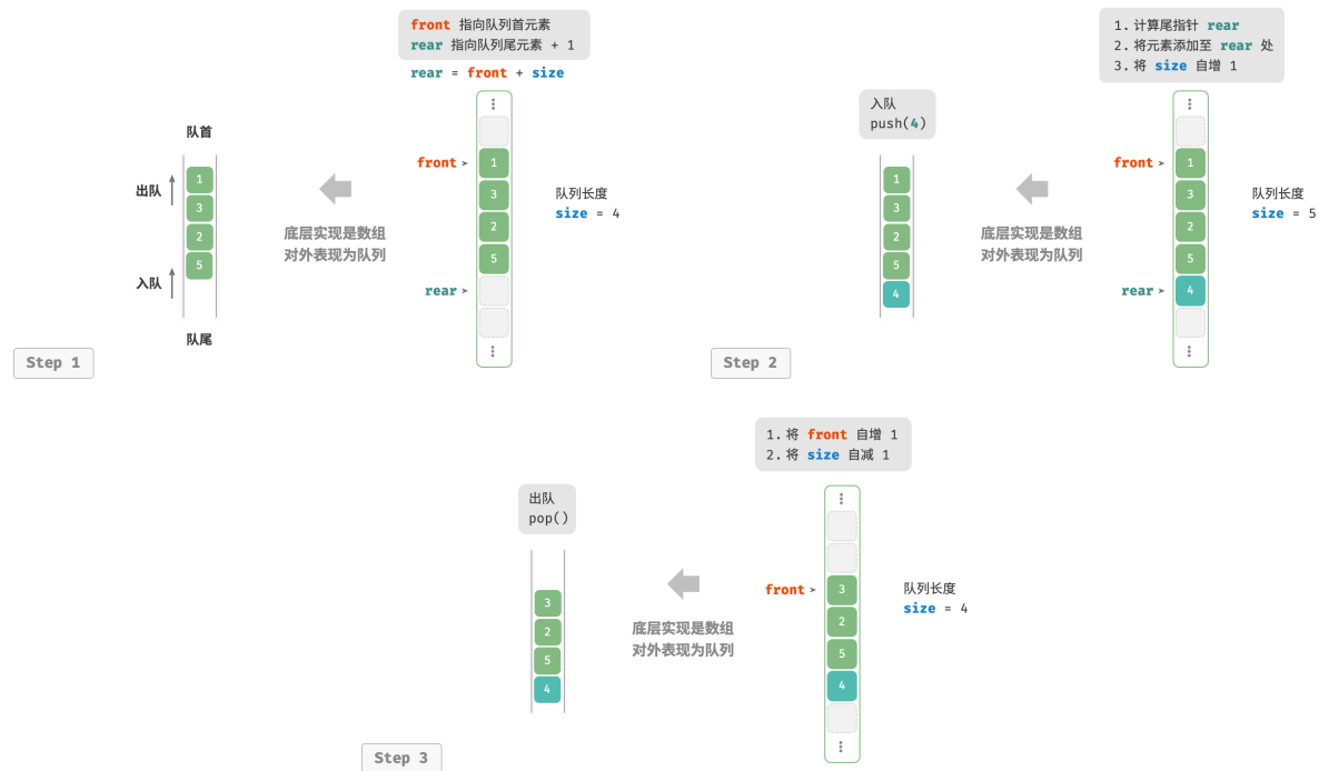
图 5-6 基于数组实现队列的入队出队操作
