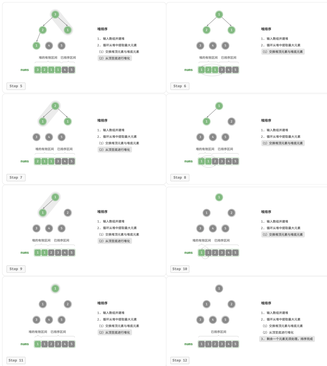
图 11-12 堆排序步骤
