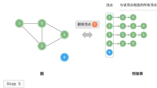
图 9-8 邻接表的初始化、增删边、增删顶点
